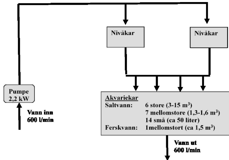
Figur 1: Flytskjema for vannforsyningen til Risør Akvarium.
