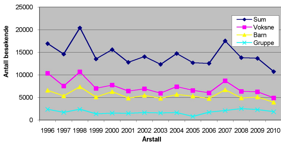
Figur 2: Antall besøkende ved Risør Akvarium i perioden 1996-2010.
