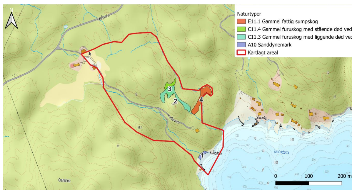
Figur 1: Kartlagt areal avmerket i rødt. Naturtyper iht. instruksen avmerket i egne polygon.
